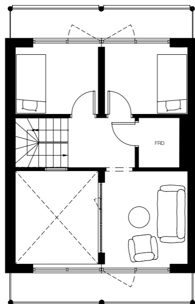
Hustyp A1, plan 2
